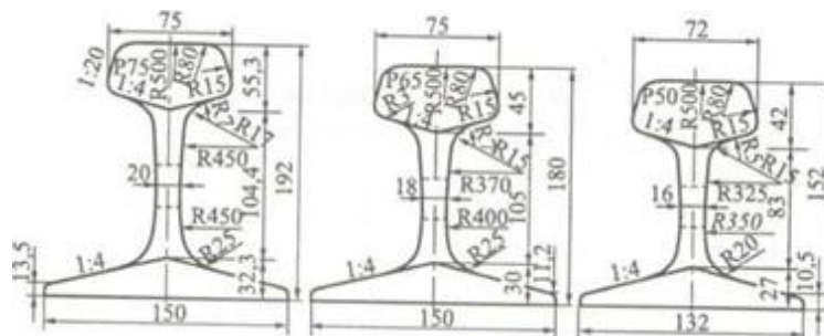
Рис. 1. Основные типы рельсов
