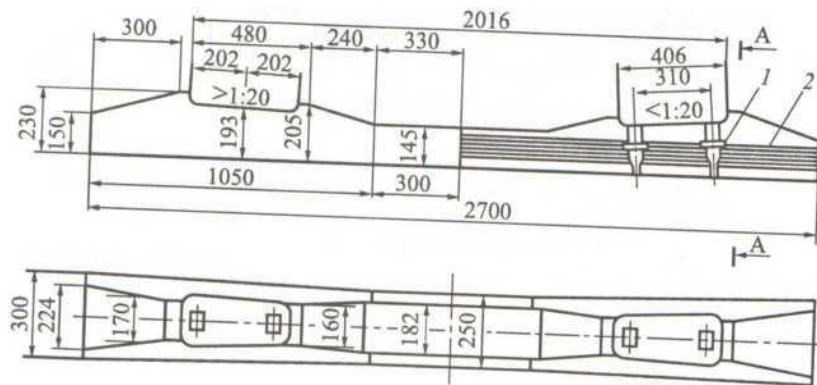
Рис. 9. Железобетонная шпала типа III
